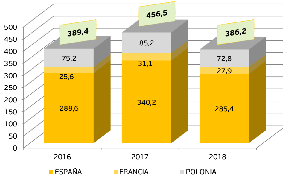
Producción (GWh)
